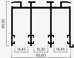
Perfil superior 3 carriles Iras 070369
