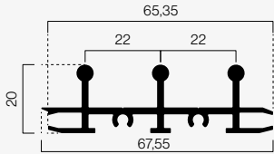
Perfil inferior 3 carriles Iras 070370
