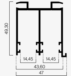
Perfil superior 2 carriles Iras 070380
