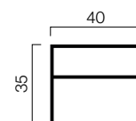
Soporte estructural 35x40 aluminio doble 051384
