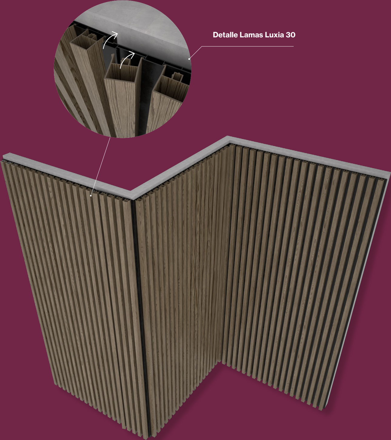
Ejemplo de instalación de 3 muros contiguos en caso de haber esquinas exteriores e interiores.
