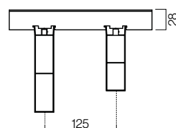
Lama Luxia-90 y 120 combinadas Paso 8 • 8 lamas/ml
