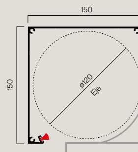
Perfil registro 150 024463
