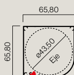
Perfil cajón 65 100162
