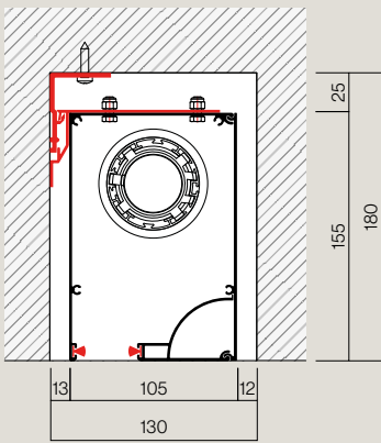
Espacio mínimo para la instalación del cajón en nicho
