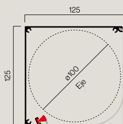
Perfil registro 125 Dante 024972
