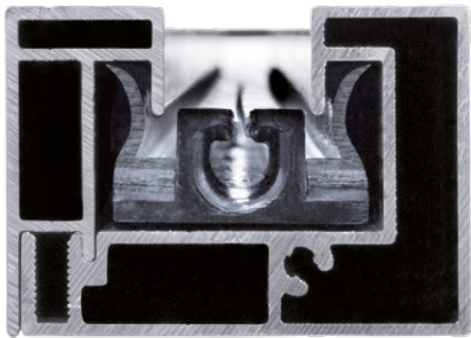
Perfil guía de coextrusión.
